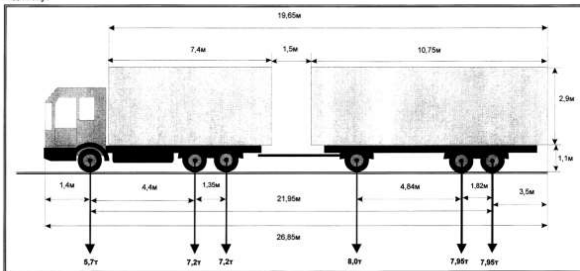
СХЕМА транспортного средства (автопоезда), с использованием которого планируется осуществлять перевозки тяжеловесных и (или) крупногабаритных грузов, с указанием размещения такого груза
